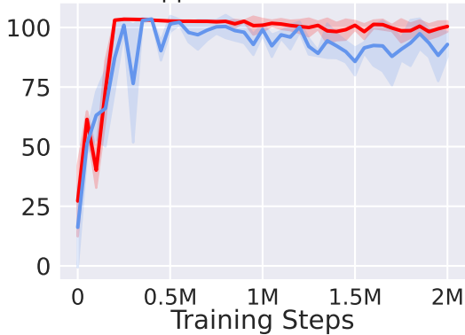
hopper-medium-v2-v2
