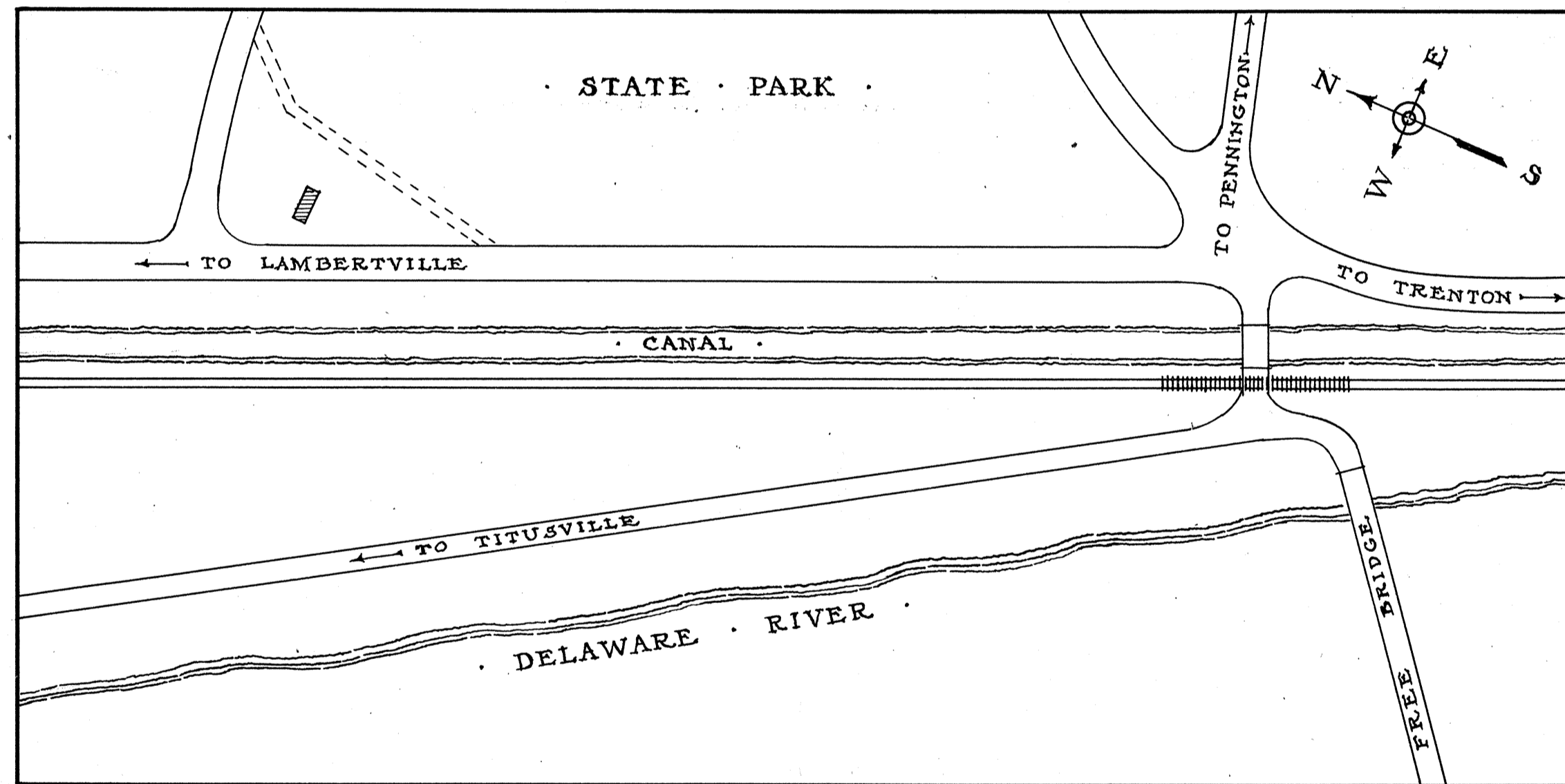
· PLOT · PLAN · SCALE 1"=200'
